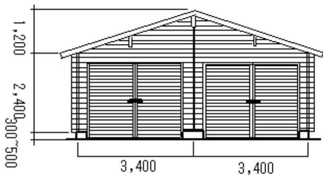
正面図
